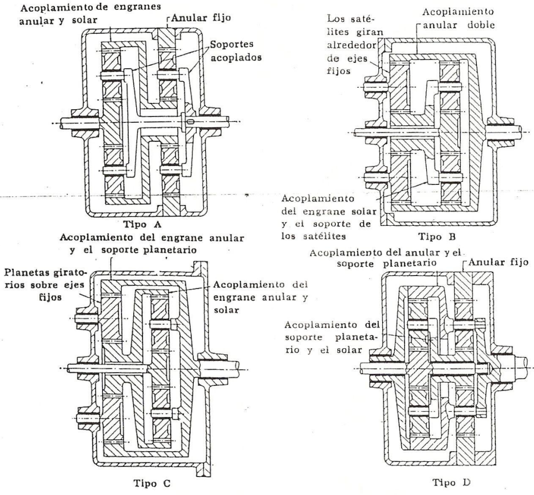
FIG. 3-17. Algunas disposiciones esquemáticas de engranajes epicicloidaes acoplados
